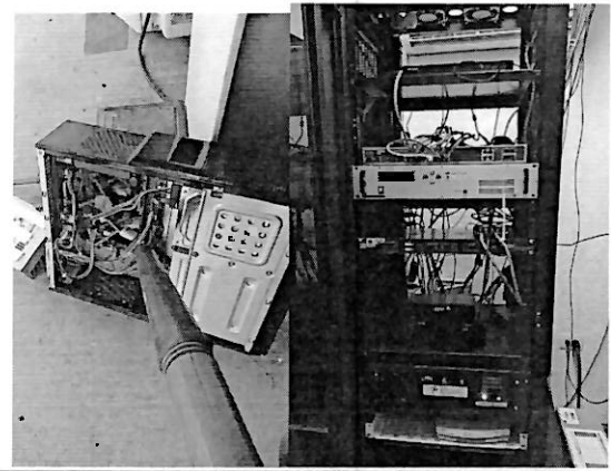
Limpieza de los cpus de computadoras, y del rack de equipos en los estudios y oficinas.
