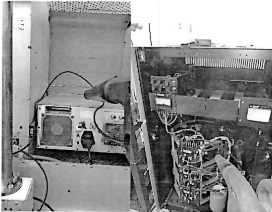
Mantenimiento limpieza al transmisor y regulador de voltaje
