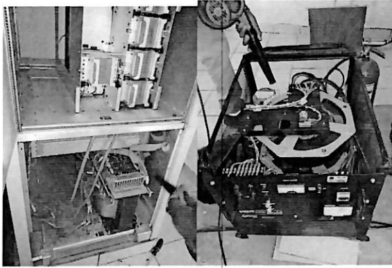
Limpeza del transmisor de FM y regulador de voltaje en cuarto de transmisión
