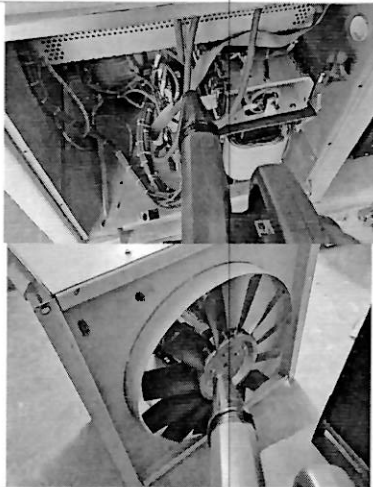
Mantenimiento y limpieza al transmisor, fuente de poder y motor-ventilador del transmisor
